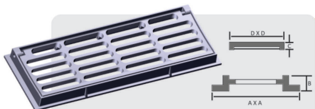
Grelha Articulada GR-135 Cód.: 11184 | B-125
